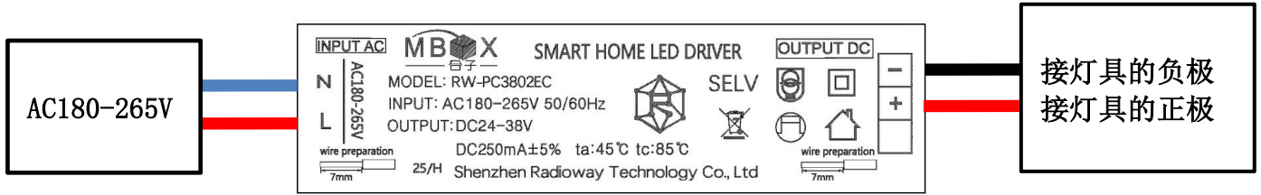
单色温调光驱动器
