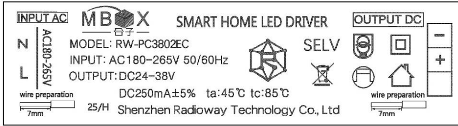
单色温调光驱动器
