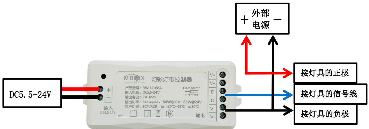
RW-LC168A 接“外部电源+” “外部电源-” “输出 D” “输出 V-”
